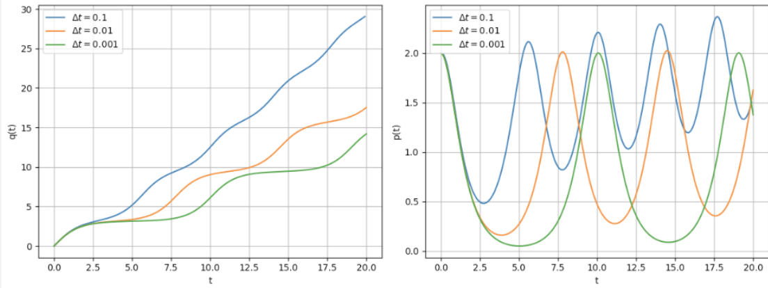
Figure 2: Evolução temporal do momento canônico p(t) usando o Método de Euler Convencional.
